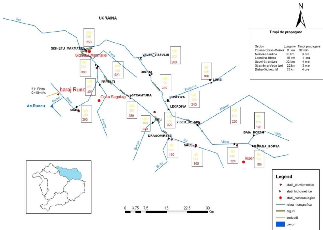
e) Schema de gospodărire a apelor existentă în bazinul hidrografic Tisa Superioara
