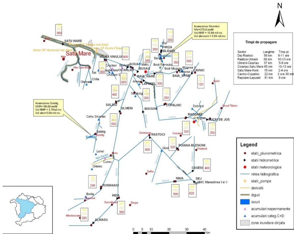
b) Schema de gospodărire a apelor existentă în bazinul hidrografic Someșul Inferior
