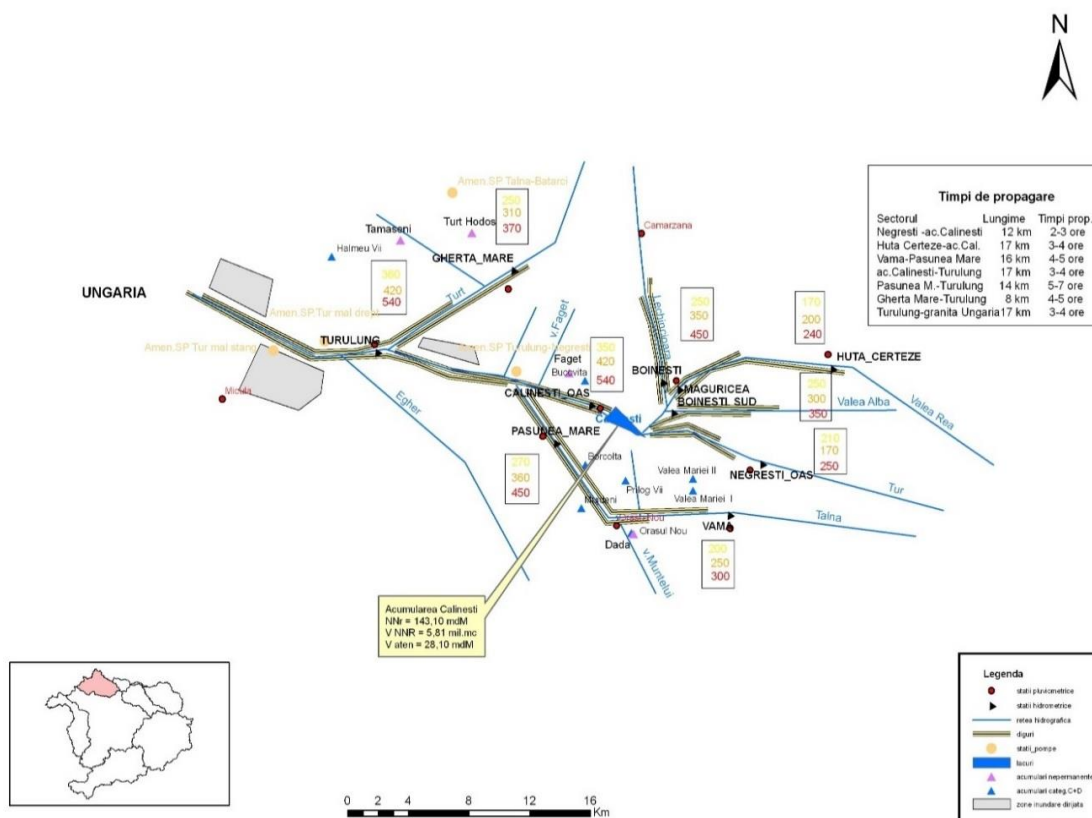
f) Schema de gospodărire a apelor existentă în bazinul hidrografic Tur
