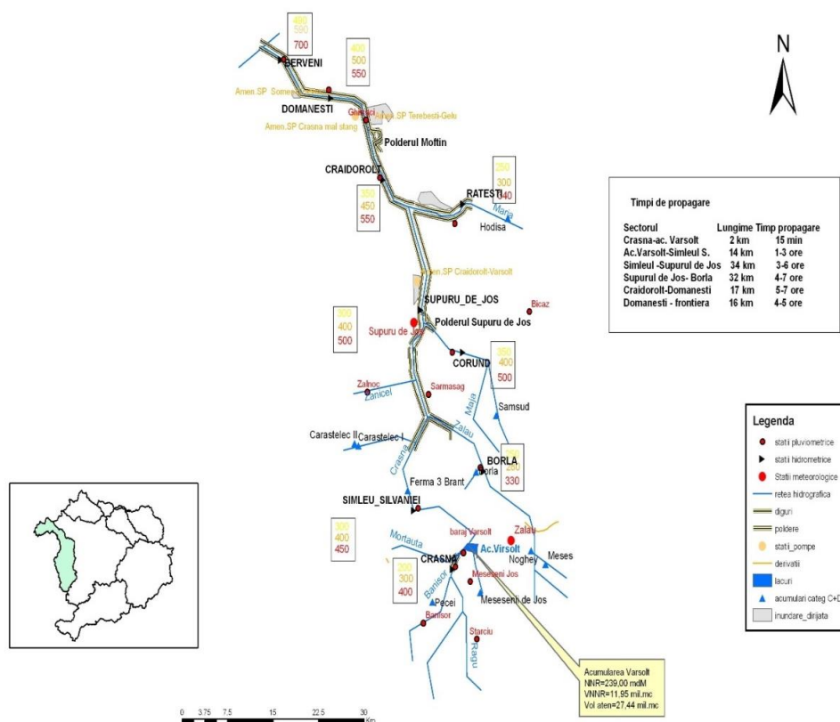
a) Schema de gospodărire a apelor existentă în bazinul hidrografic Crasna
