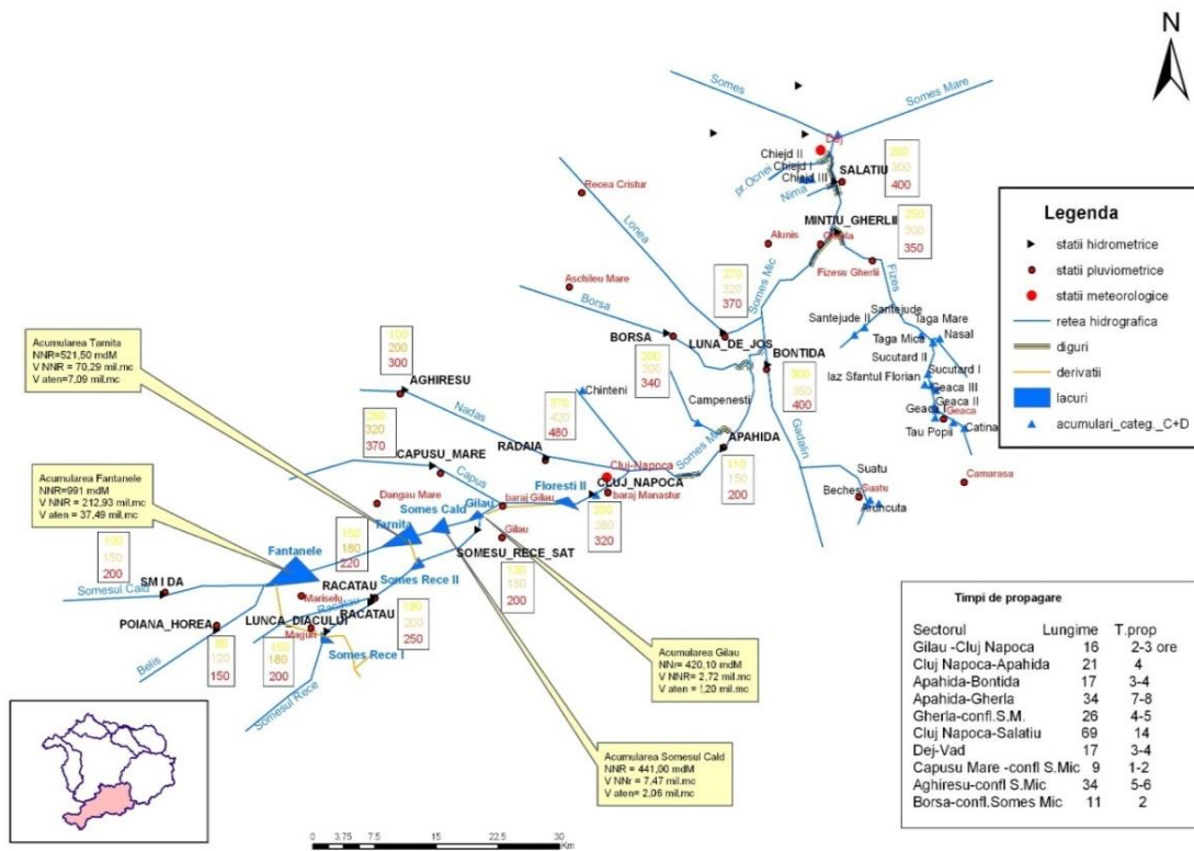
d) Schema de gospodărire a apelor existentă în bazinul hidrografic Someșul Mic
