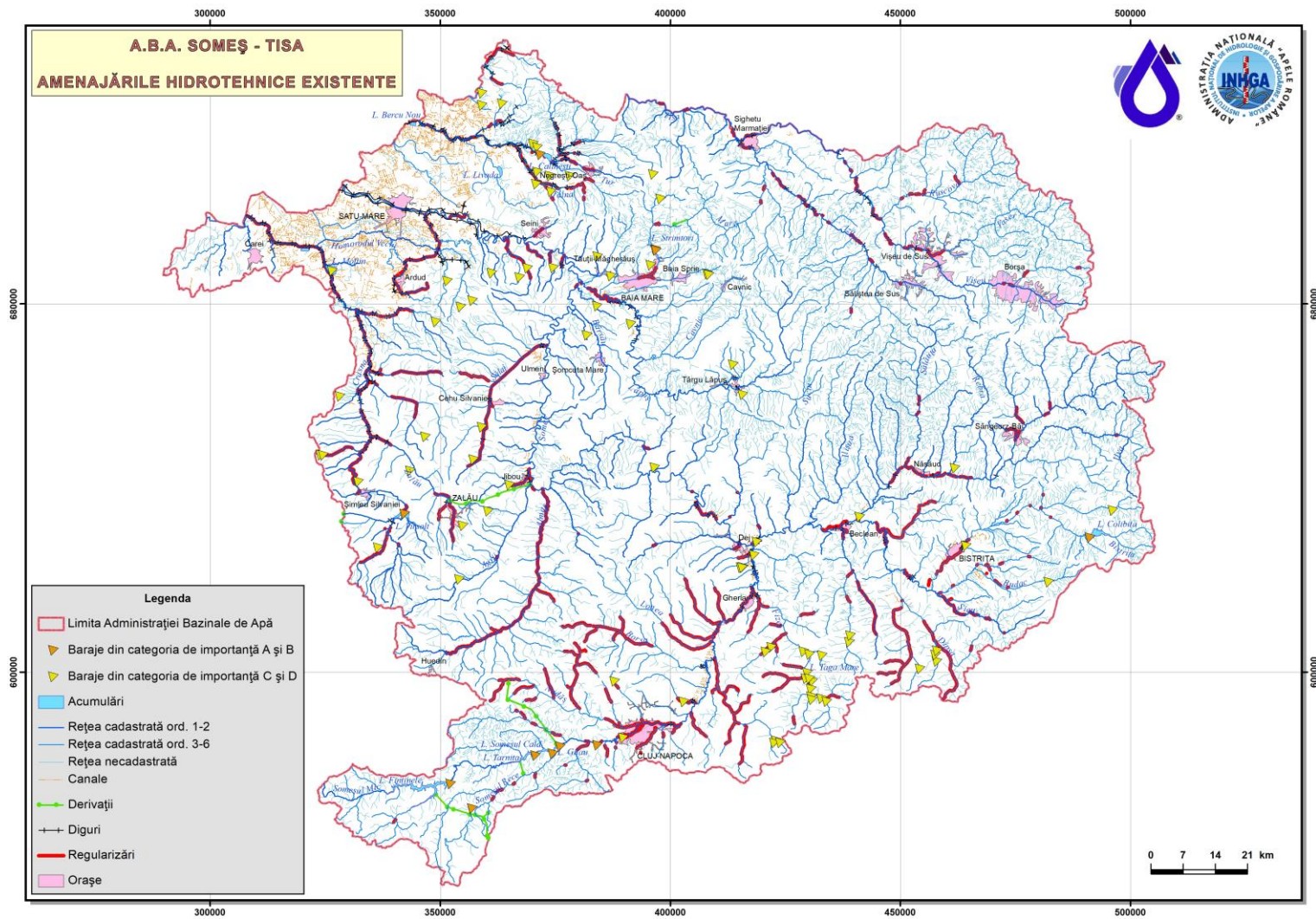
Figura 6.7.2. Amenajări hidrotehnice existente la nivelul A.B.A. Someș - Tisa
