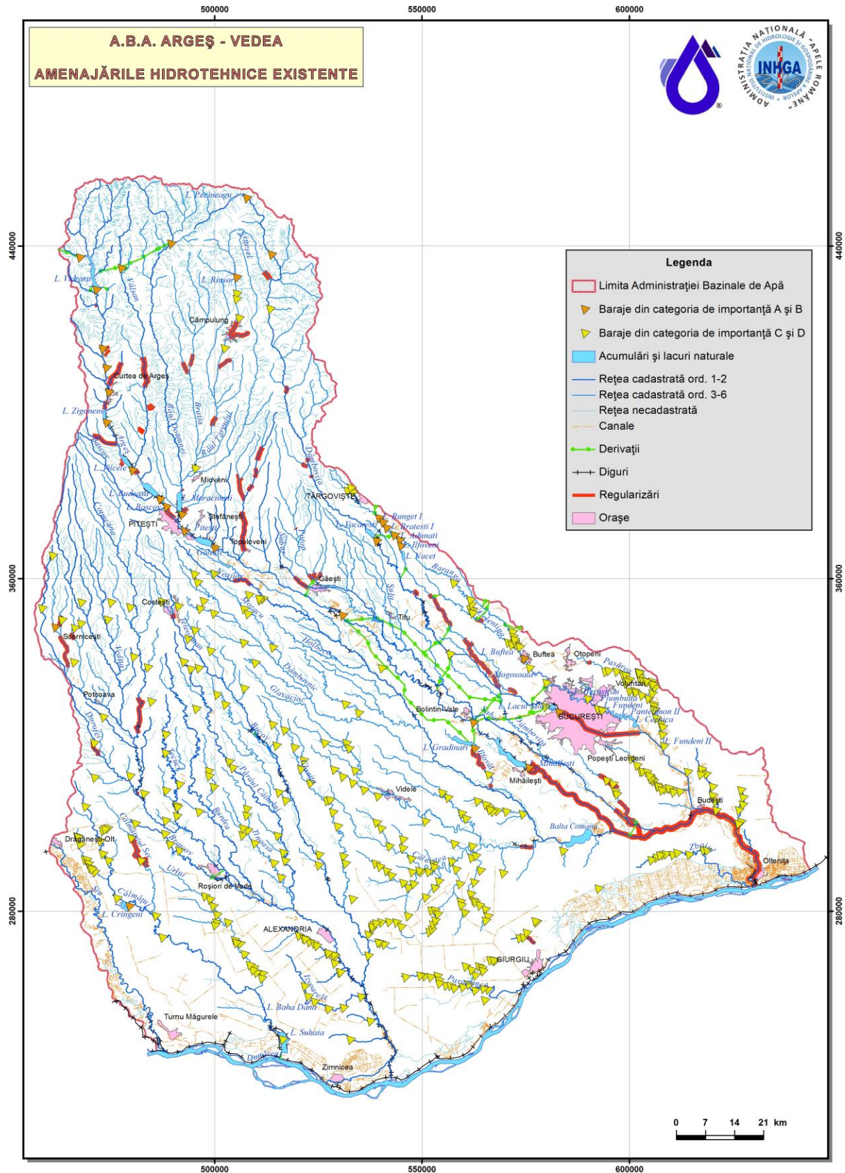
Figura 3.4.2 Amenajări hidrotehnice existente la nivelul A.B.A. Argeș - Vedeș
