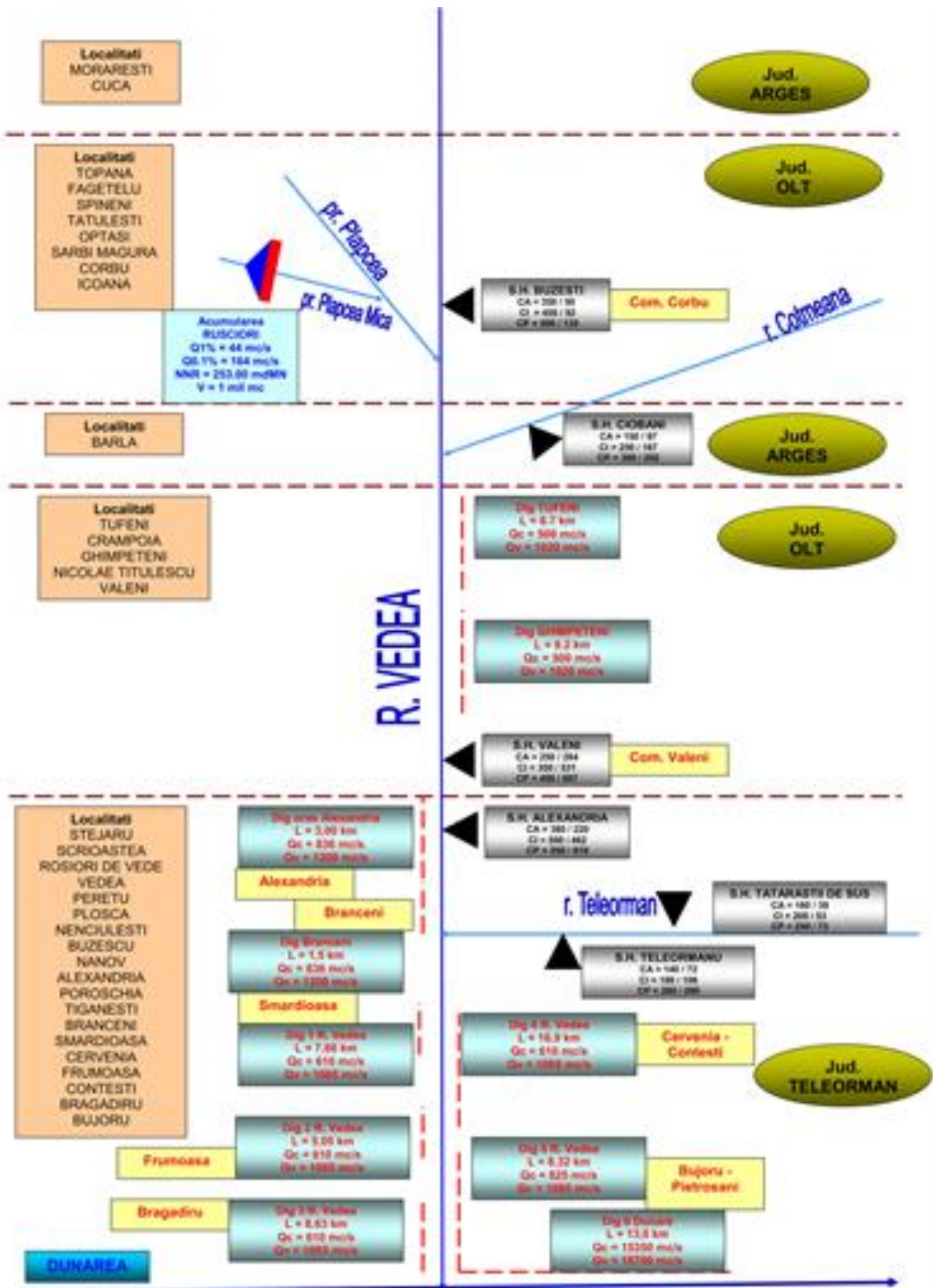
a) Schema de gospodărire a apelor existentă în bazinul hidrografic Vedeia
