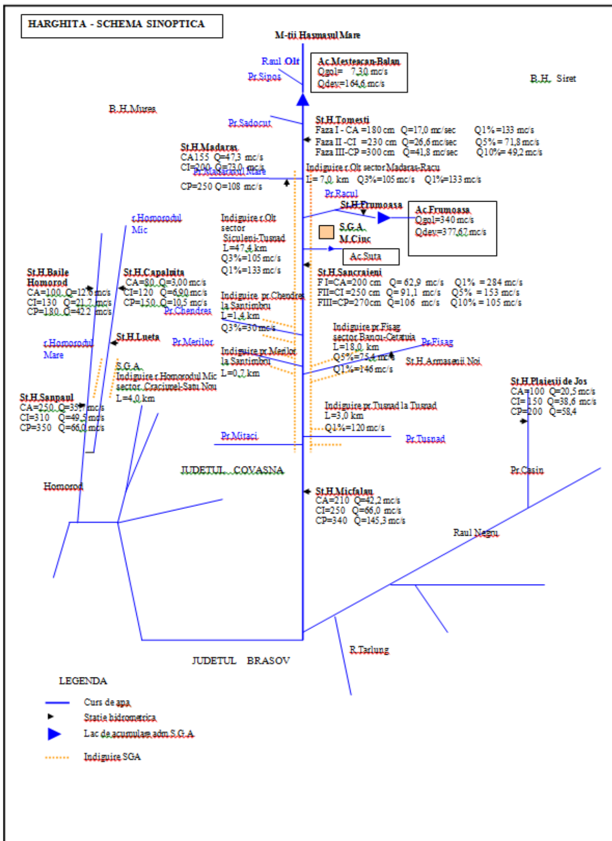
Figura 3.7.2 Schema de gospodărire a apelor existentă în bazinul hidrografic Olt, în județul Harghita
