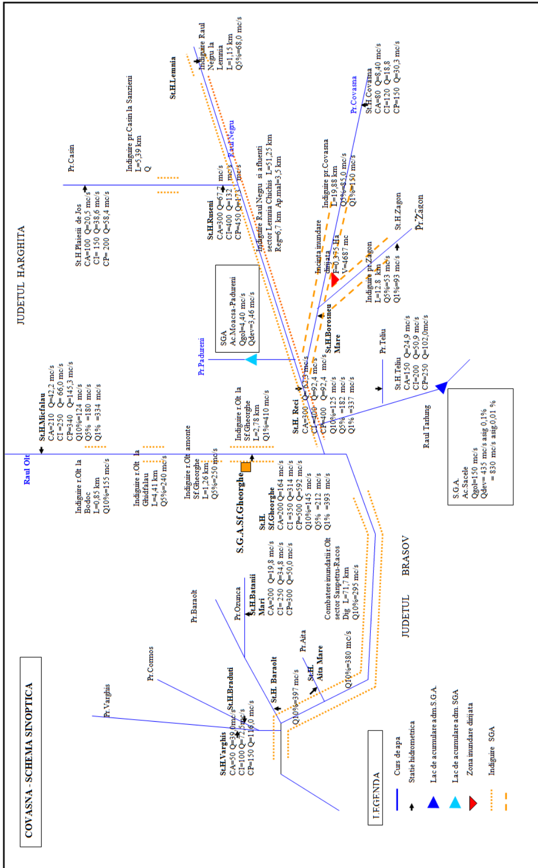
Figura 3.7.3 Schema de gospodărire a apelor existentă în bazinul hidrografic Olt, în județul Covasna
