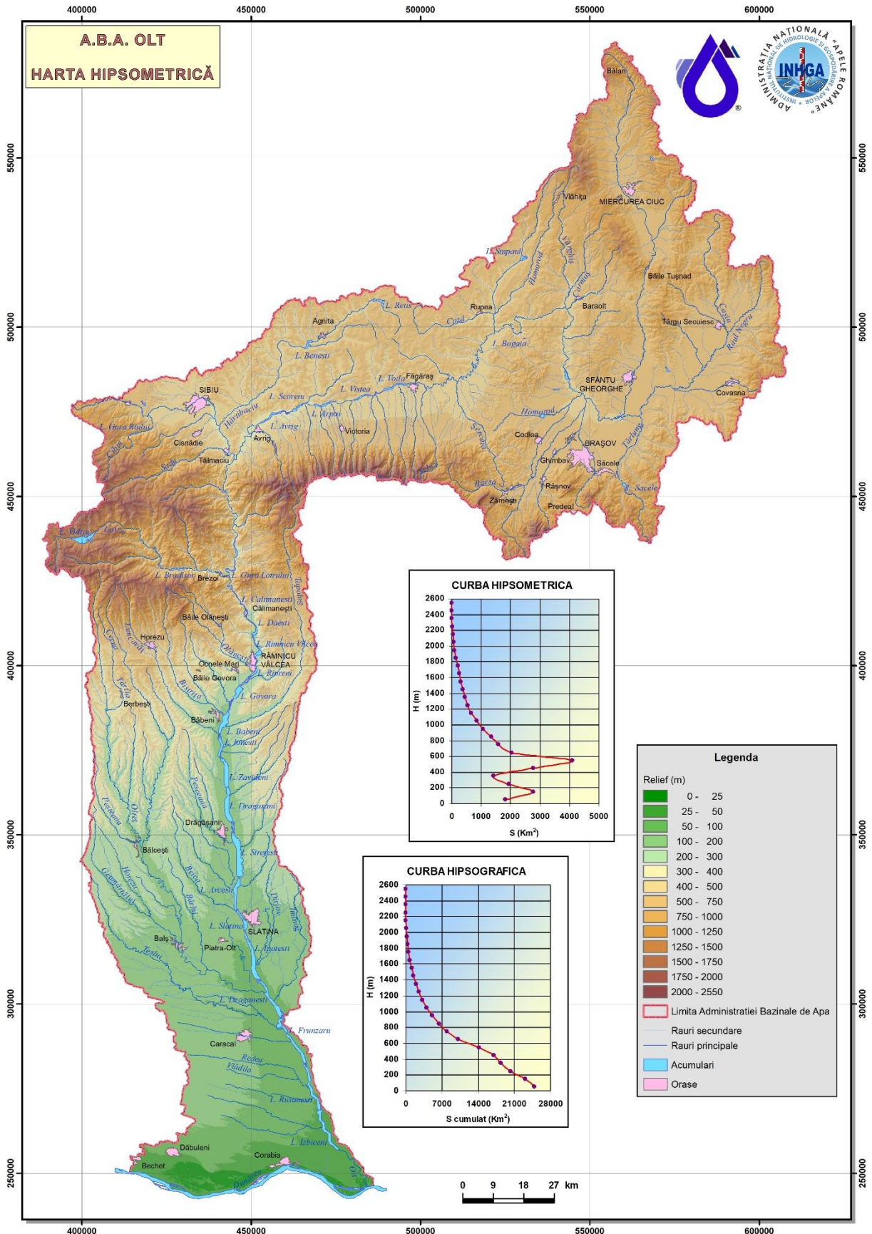
Figura 3.1.1 Harta hipsometrică la nivelul A.B.A. Olt
