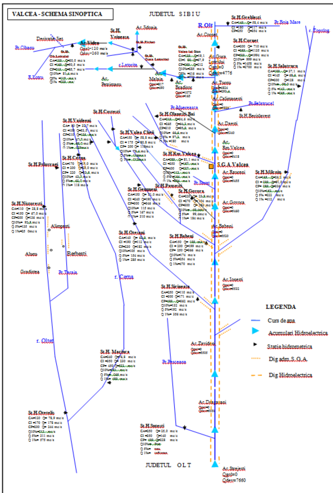
Figura 3.7.6 Schema de gospodărire a apelor existentă în bazinul hidrografic Olt, în județul Vâlcea
