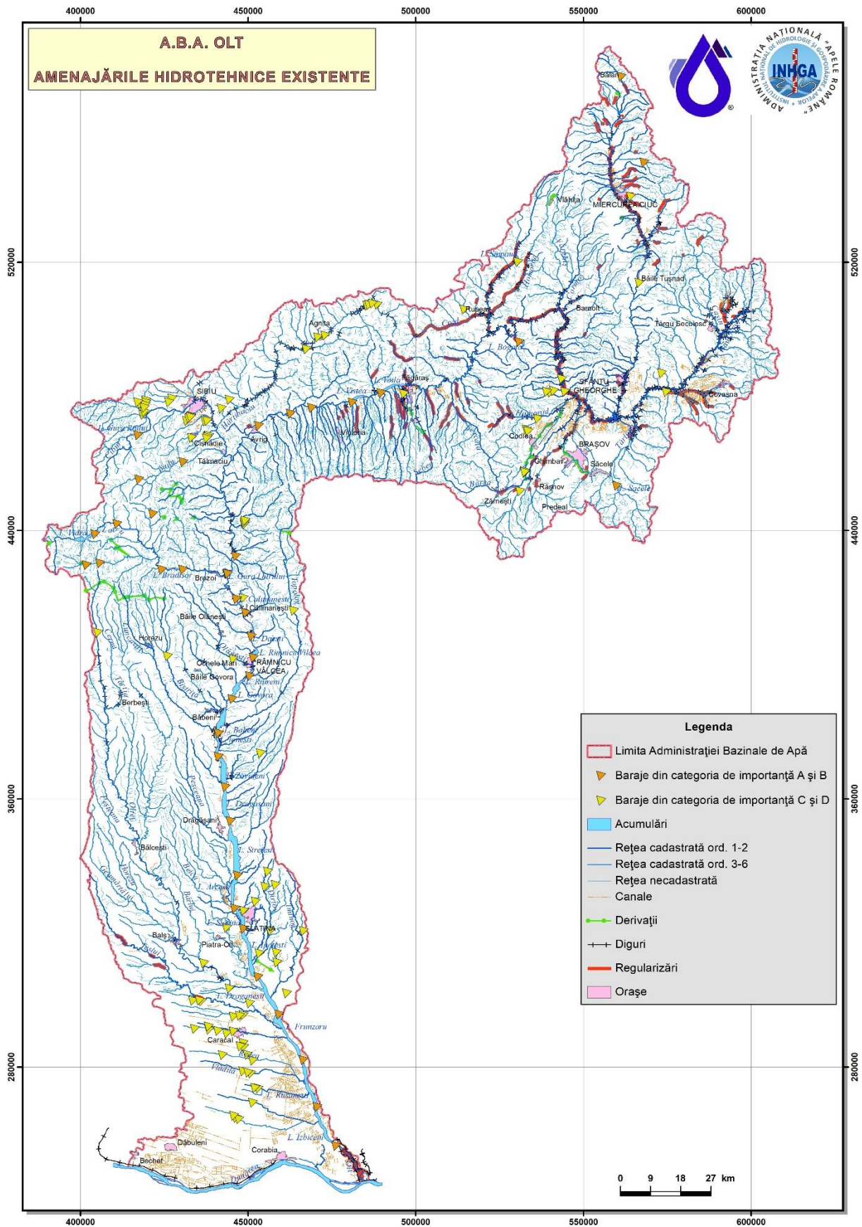
Figura 3.7.1 Amenajări hidrotehnice existente la nivelul A.B.A. Olt
