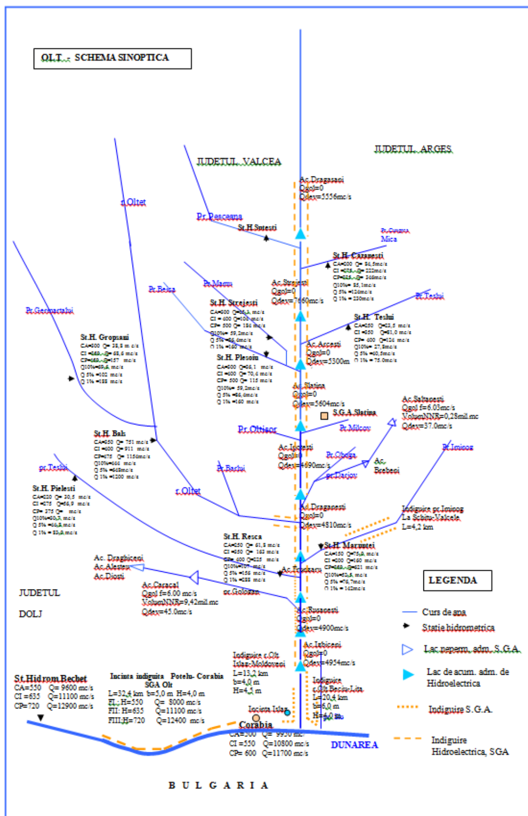
Figura 3.7.7 Schema de gospodărire a apelor existentă în bazinul hidrografic Olt, în județul Olt
