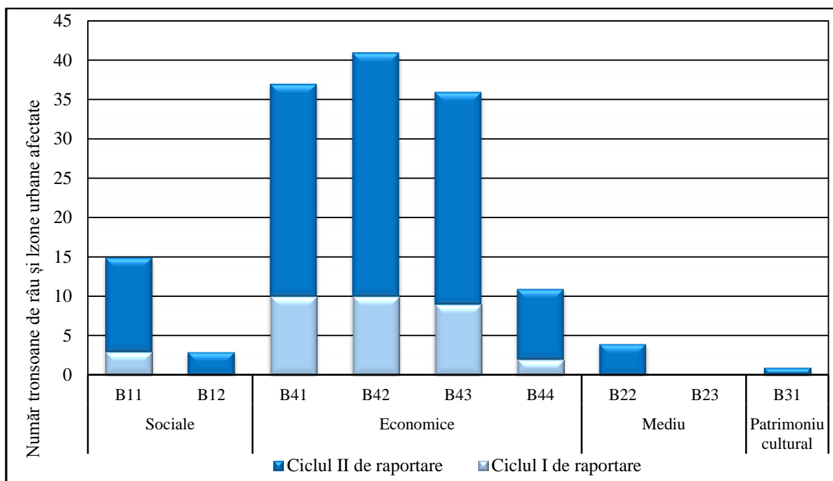
Figura 5.2.1. Tronsoane de râu și zone urbane afectate de inundații pe categorii de consecințe pentru evenimentele istorice semnificative din ciclurile I și II de implementare a Directivei Inundații 2007/60/CE la nivelul A.B.A. Jiu
