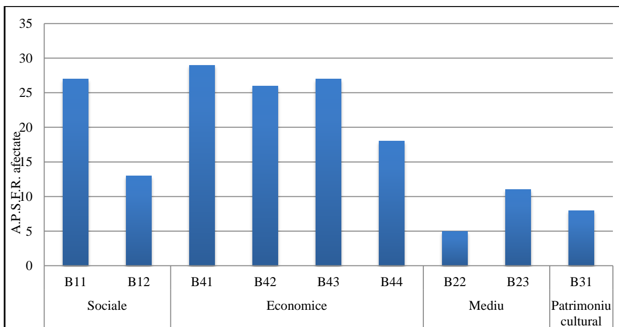
Figura 6.1 Numărul de A.P.S.F.R. raportate în ciclul II pentru care au fost evaluate categoriile de consecințe
