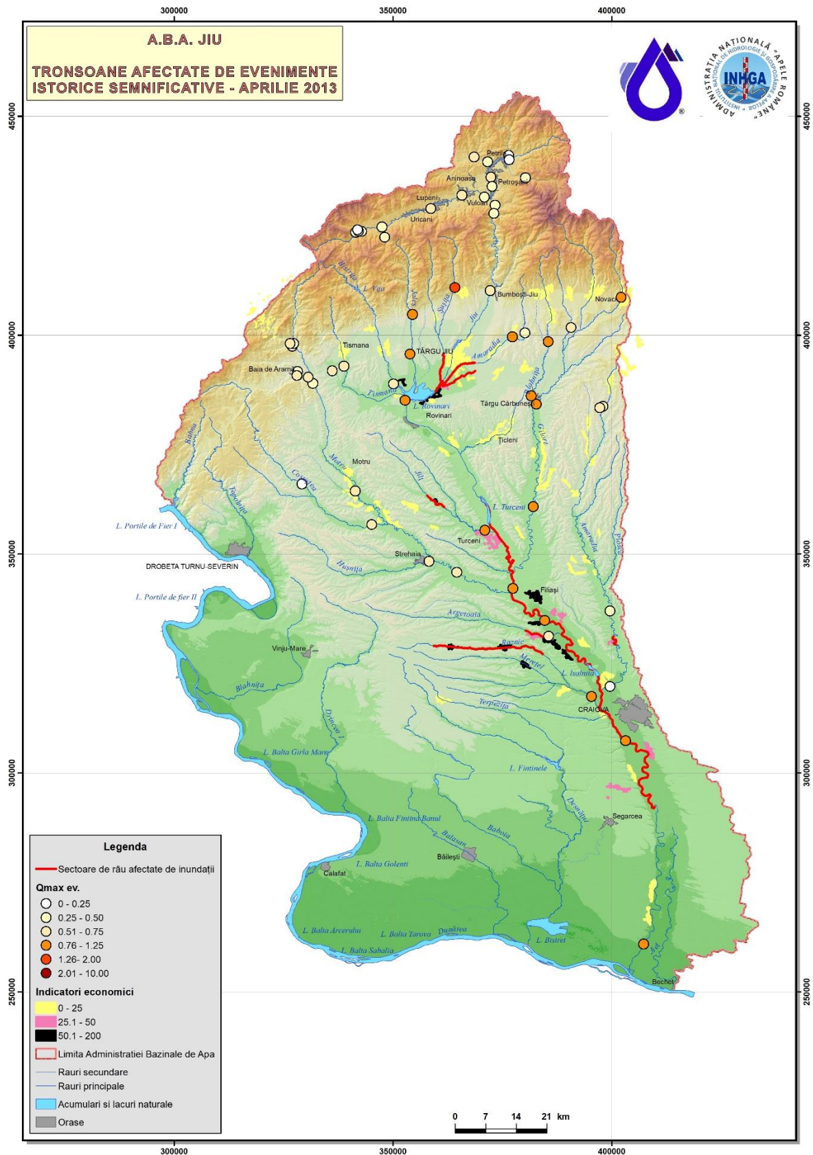
Figura 4.2.1.3 Tronsoane de râu afectate de evenimentul istoric semnificativ aprilie 2013 identificat prin analiza corelată a criteriilor legate de pagube și a criteriilor hidrologice - A.B.A. Jiu
