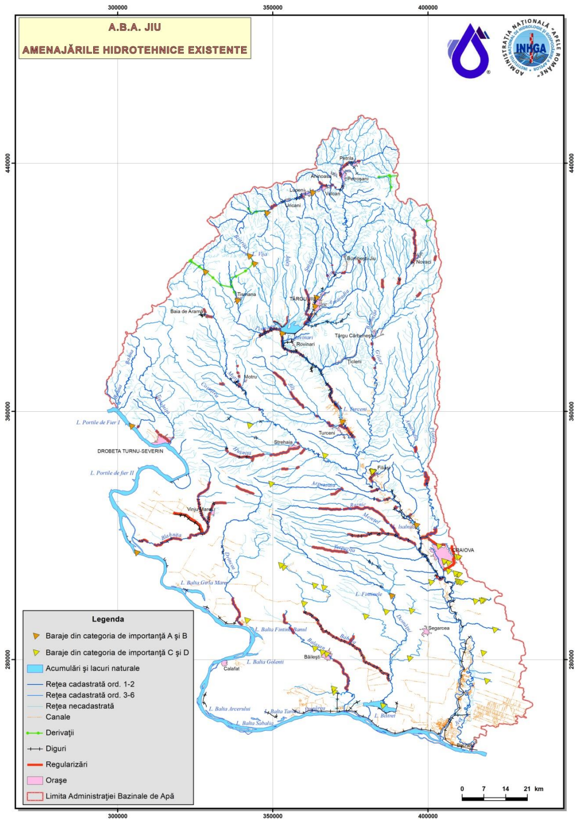
Figura 3.7.1 Amenajările hidrotehnice existente la nivelul A.B.A. Jiu
