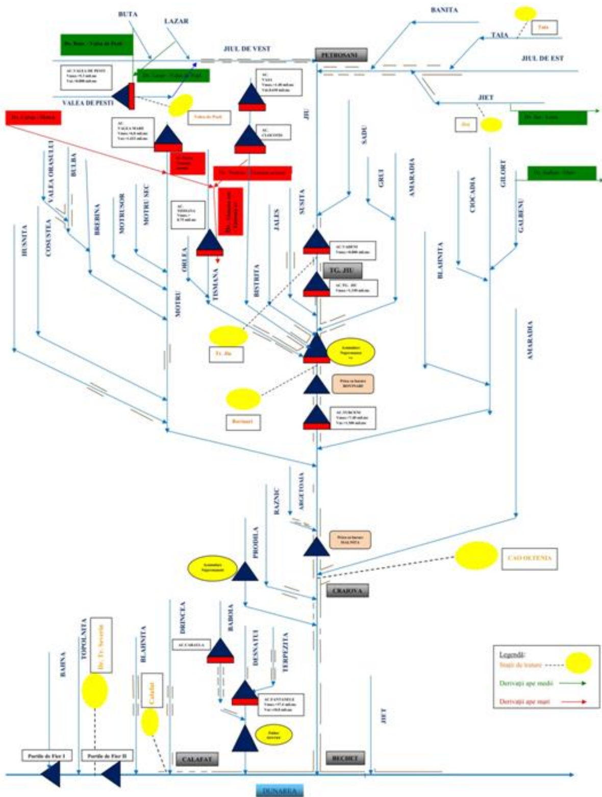
Figura 3.7.2 Schema de gospodărire a apelor existentă în bazinul hidrografic Jiu
