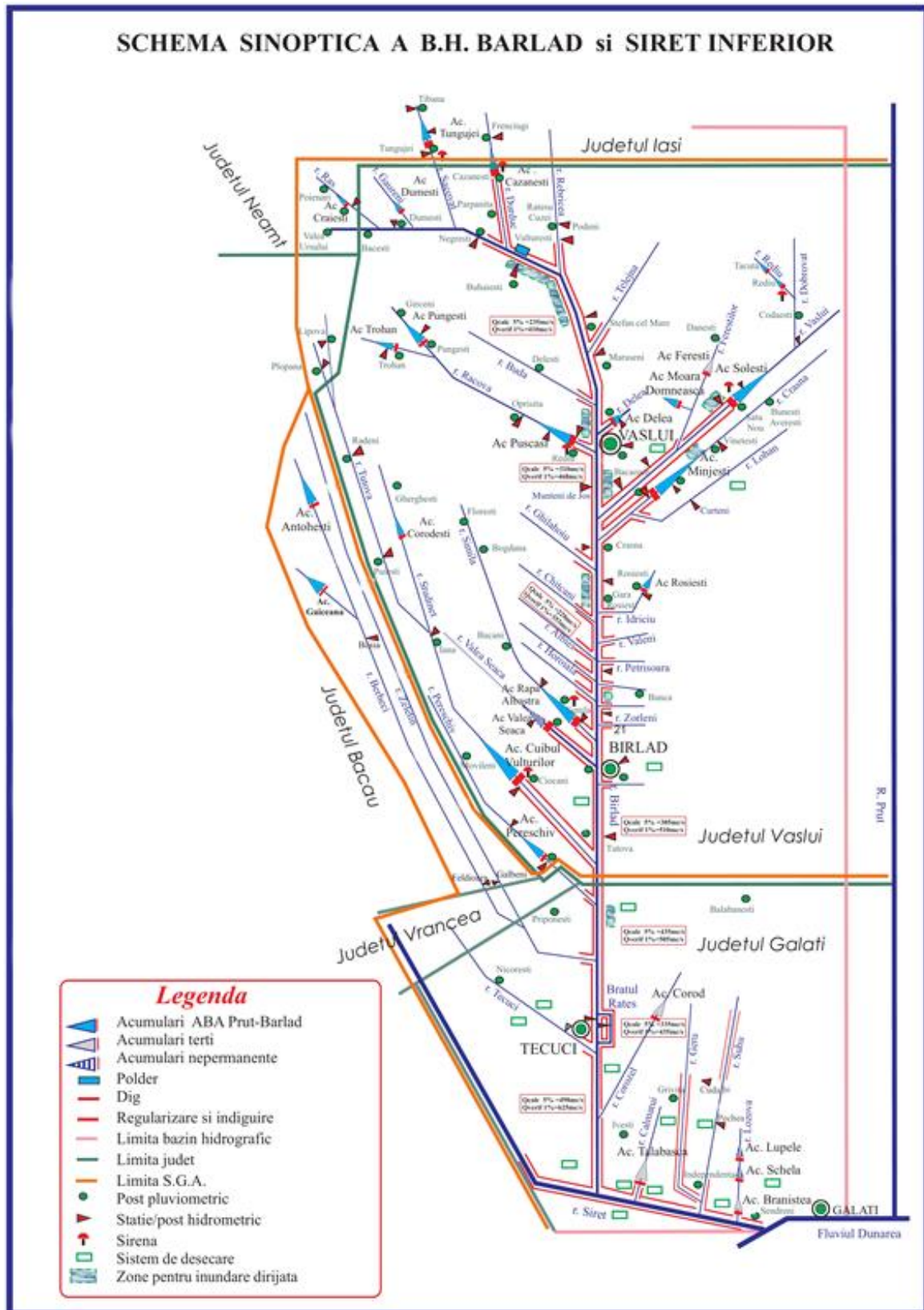
Figura 3.7.3 Schema de gospodărire a apelor existentă în bazinele hidrografice hidrografice Bârlad și Siret inferior
