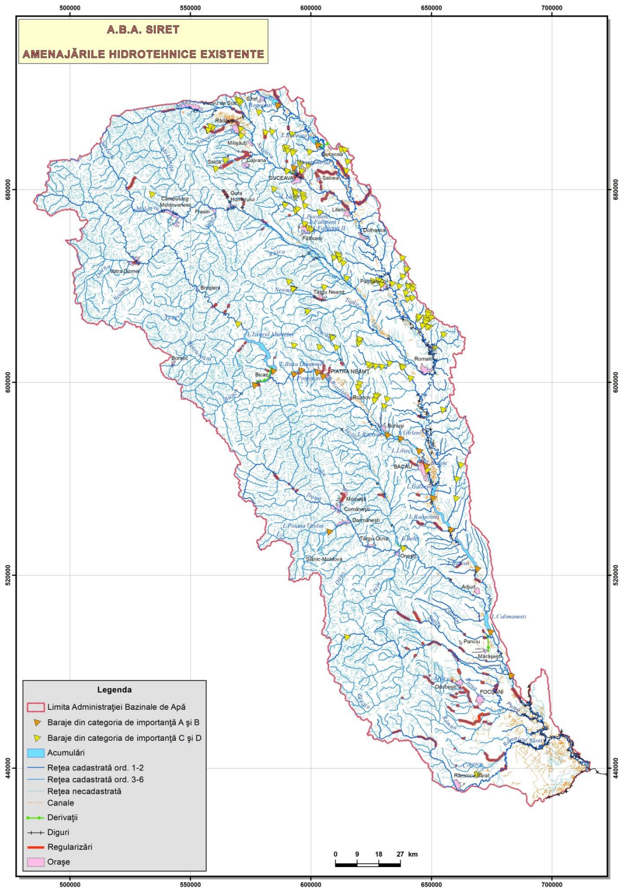
Figura 3.7.1 Amenajări hidrotehnice existente la nivelul A.B.A. Siret
