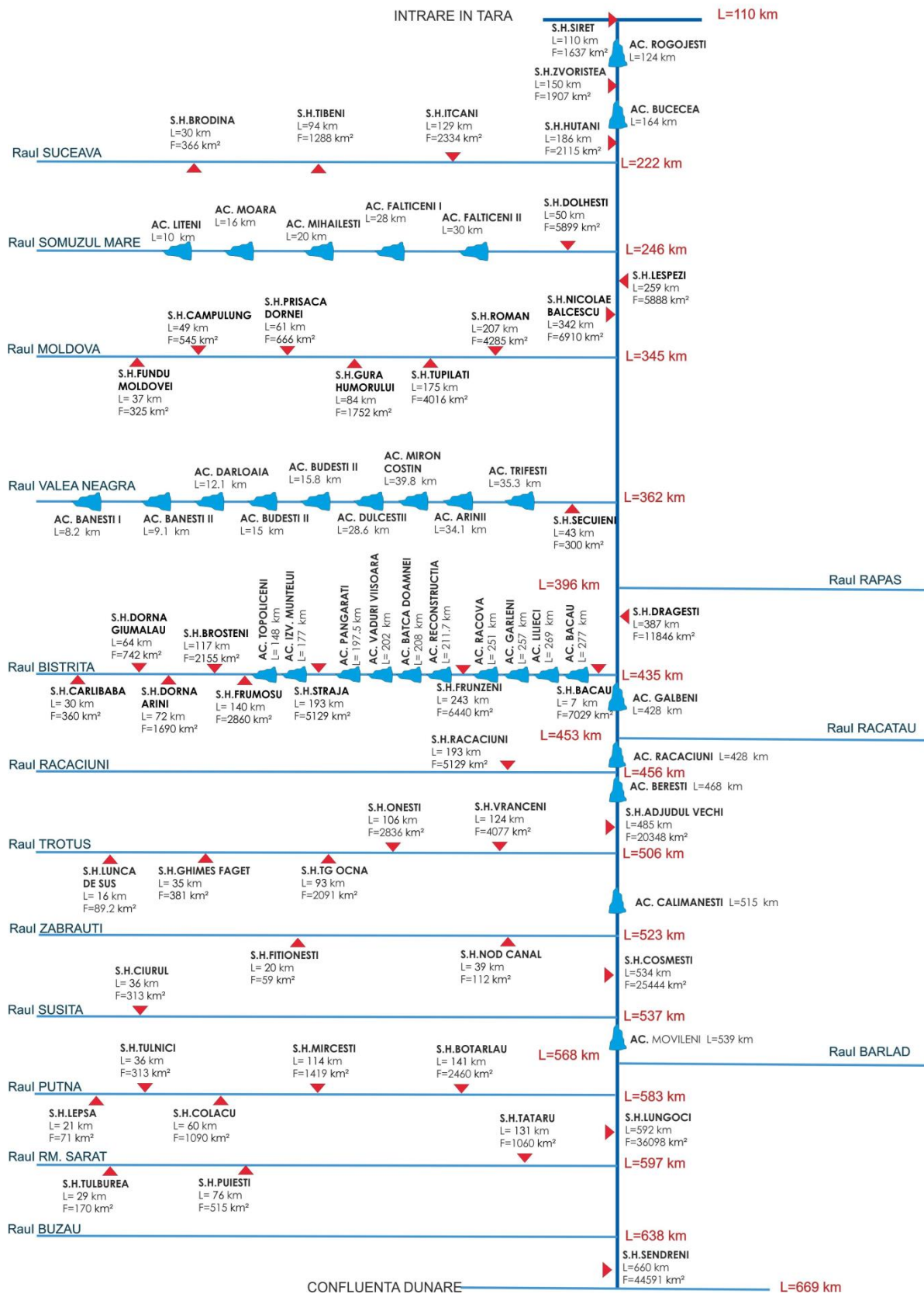
Figura 3.7.2 Schema de gospodărire a apelor aferentă spațiul hidrografic Siret
